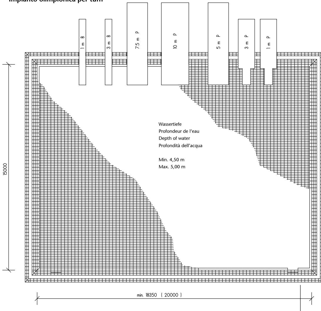
Draufsicht/Vue d'en haut/Top view/Vista dall' alto
